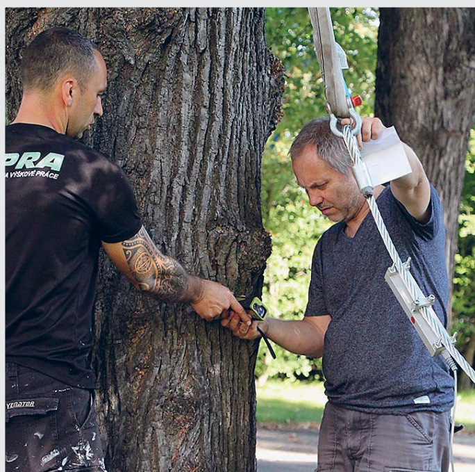
Tahové zkoušky jsou nejkomplexnější metodou pro zjištění stability stromu. Foto: Dita Círová
